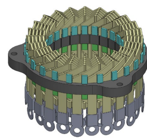
提案構造アルミニウム巻線を備えた EV 用高速モータの 3D モデル
