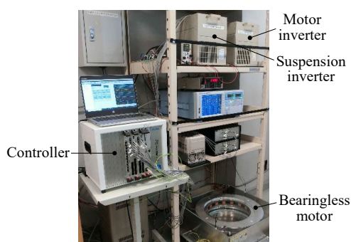
半導体製造装置用ベアリングレスモータの実験装置
