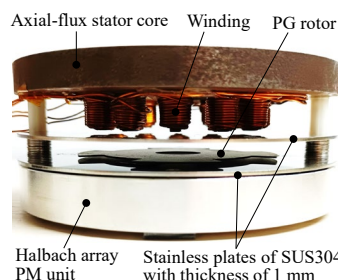
反磁性グラファイト板を用いた革新的グラファイトモータ
